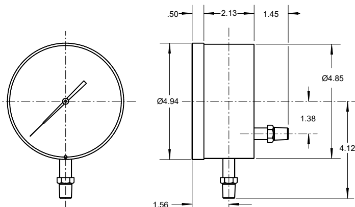
4.5" No Flange
